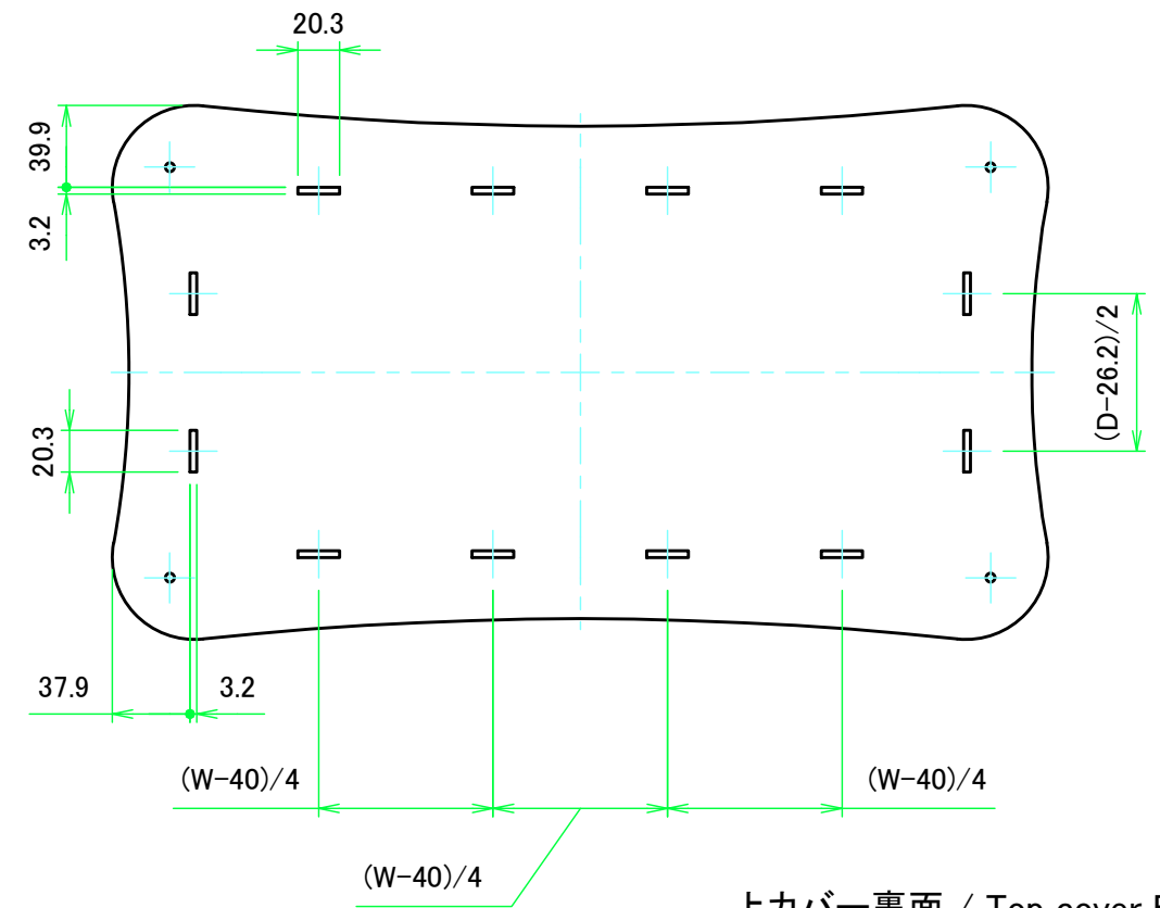
上カバー裏面 / Top cover Backside
